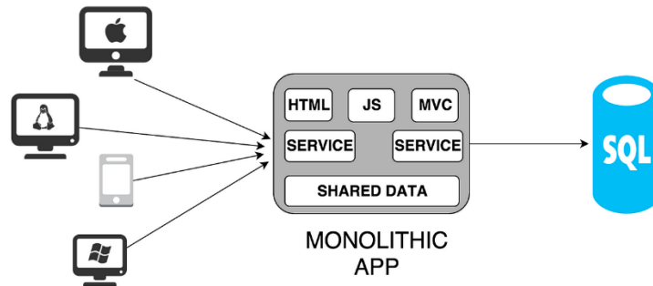
Gambar 3. 3 Model Arsitektur Monolithic
