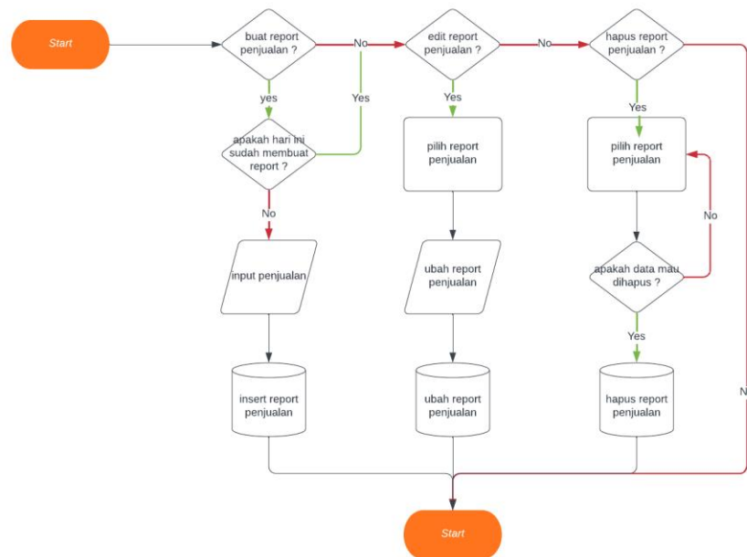
Gambar 3. 7 Diagram alir report penjualan
